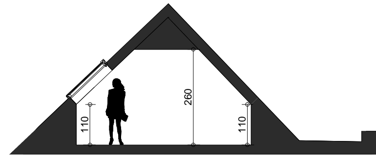
principe snede zolder
