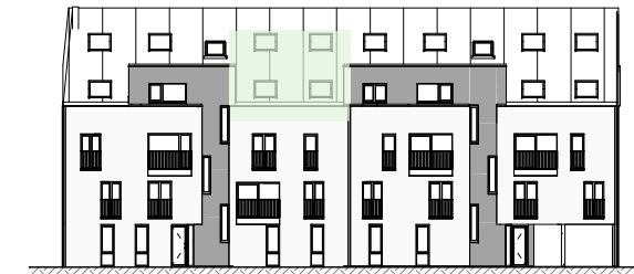
voorgevel
