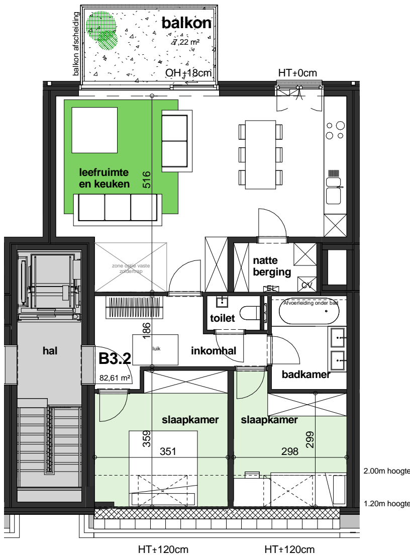
verdieping 3
