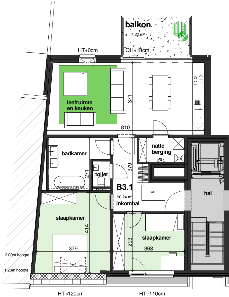
verdieping 3
